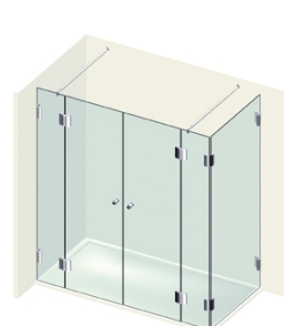
2 fix üvegről nyíló ajtó, 3 fix üveggel
